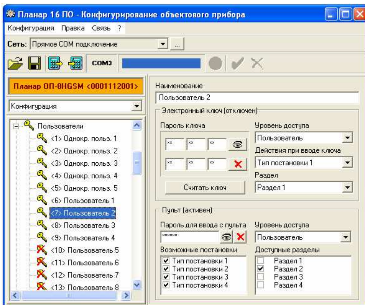
Рис. 12.18 Список пользователей
